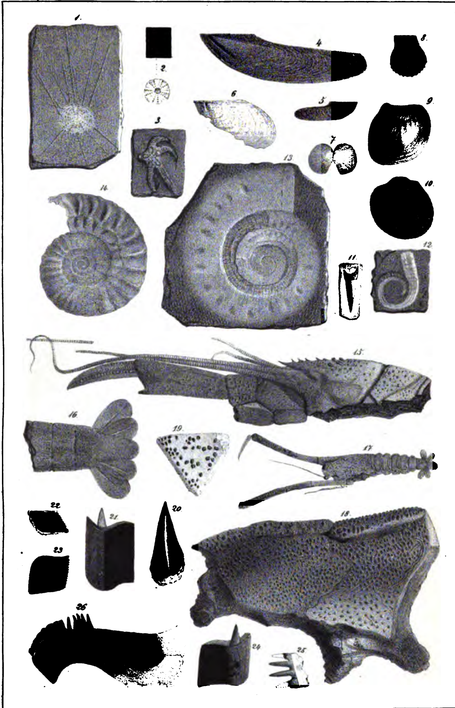
Quenstedt, Jura.
